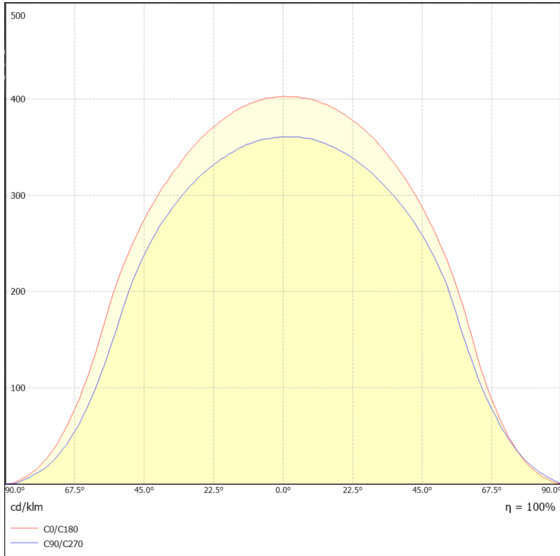
CURVA ILUMINACIÓN - DISTANCIA
