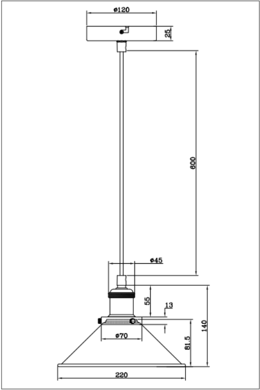
DISEÑO TÉCNICO (mm) INDUSTRIAL
